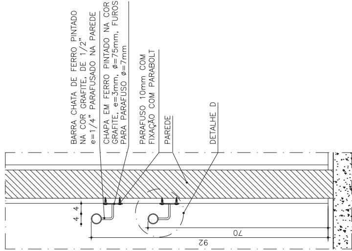
CORRIMÃO FIX. PAREDE SEÇÃO VERTICAL
