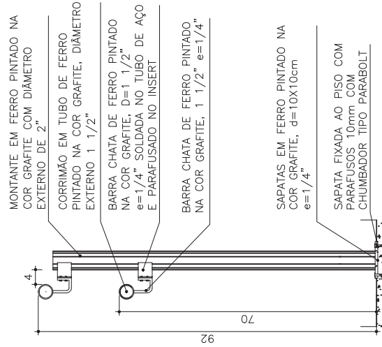
CORRIMÃO FIX. MONTANTE SEÇÃO VERTICAL
